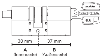
GERDA SLR Modularzylinder - minimale Länge
