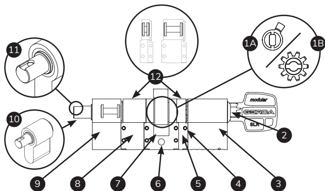
GERDA SLR Modularzylinder
