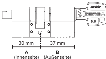
GERDA SLR Modularzylinder - minimale Länge
